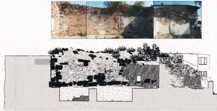
Çizim 2: 9 nolu iç kule ile 9 nolu dış kule arasında bulunan iç beden duvarının rölövesi.
