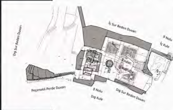
Çizim 1: Zindan rölöve planı
