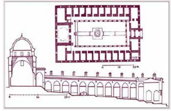
Yıldırım Darüşşifasının plan ve kesiti
